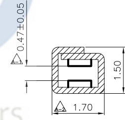
Section:E-E
