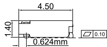
04~10 Pin
